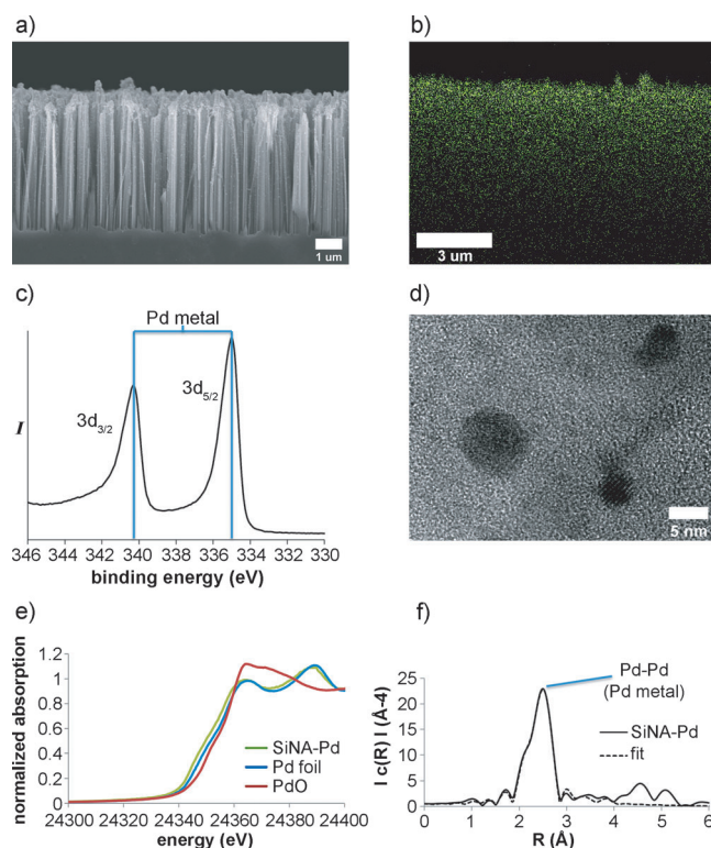
Figure 1. a) SEM, b) SEM/EDX, c) XPS, d) TEM, e) XANES, and f) FT-EXAFS of SiNA-Pd.
